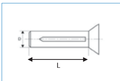
DIN 1477 - ISO 8747 - EN 28747 CTF1
